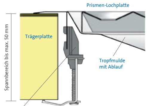
Querschnitt Trägerplatte / Einlass-Schänke
