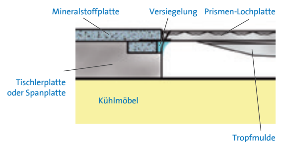
Querschnitt Trägerplatte / Unterbau-Schänke
